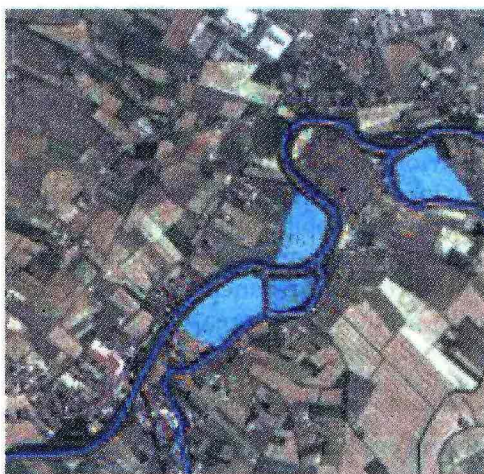
Uno studio per la laminazione delle piene del fiume Monticano alla confluenza con il fosso Borniola
